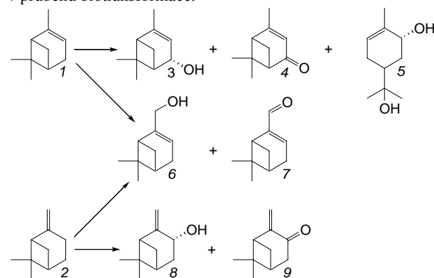
Schéma 1: Hlavní složky terpentýnu: \alpha -pinen (1), \beta -pinen (2), a hlavní produkty jeho biotransformace: trans -verbenol (3), verbenon (4), trans -sobrerol (5), myrtenol (6), myrtenal (7), trans -pinocarveol (8), pinocarvon (9)
