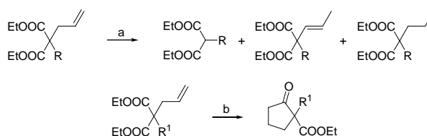
Schéma 1. a) Rh-kat. 5 mol.%, Et 3 Al 2 eq., toluen, rt. b) [Rh(PPh 3 ) 3 Cl] 5 mol.%, Et 3 Al 2 eq., toluen, rt. R 1 = benzyl, p -xylyl, 3-methyl-2-butenyl.
