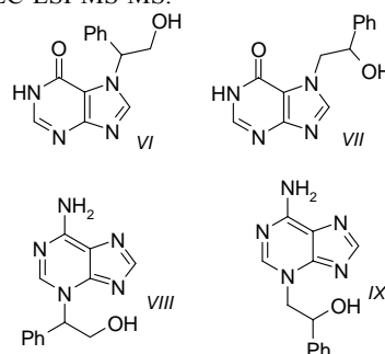
Obrázek 1. Struktury připravených aduktů DNA
