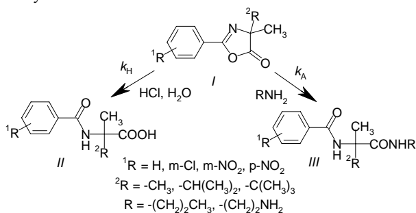
Schéma 1. Hydrolýza a aminolýza substituovaných 4-alkyl-4-methyl-2-aryl-4,5-dihydro-1,3-oxazol-5-onů
